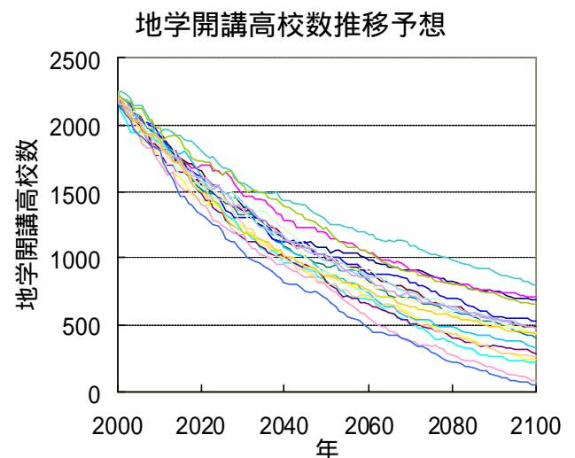
図3. 図2と同様の方法で全国の地学開講高校数の 1999 年と 2002 年のデータ（柴山，2002）を元に推移を予測したもの。図2に比べ初期値を反映して減少の程度はややゆるいように思われる。
