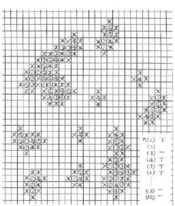
図8. 碁石モデルをプリント上で鉛筆をさいころがわりに手作業で実習した例。印は最初に仮定した破壊の種。○は隣接格子に破壊が伝播,また×は破壊伝播がストップしたことを示す。右下は破壊格子数の順に仮想地震の数を正の字を書いて集計中の様子。岡本(1997)より。
