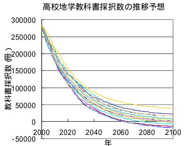
図2. 地学教科書採択数の今後の推移予測。1996年～2000年の採択実数（柴山，私信）を初期値に指数減衰近似+5%ランダム変動を加味した予測の20試行分。
