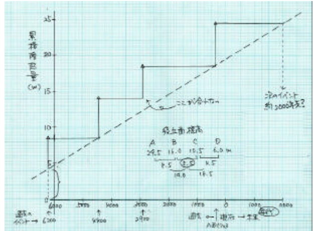
図 16．時間予測モデルのグラフ化の例：上記地形図から読み取った段丘面の高さより、過去の地震での隆起量を計算。過去の地震の年代を横軸に、累積隆起量を縦軸にとった階段上のグラフ。これから、次の地震の再来時期をおおよそ推測することができる。図15で段丘面の高さの読み取りをどうするかで、上図のように合わない部分がでたりする。
