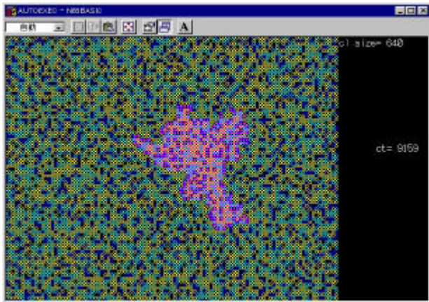
図12 PC画面上の砂山モデル.色の違いが状態量の違いを示す．中央の塊が破壊が生じた区画．ときどき画面全体に波及するようなシステムサイズの地震が起こるのが興味深い．今は時代遅れとなった感のあるN88BASICによる実行例である．
