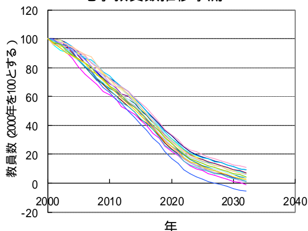
図5. 東京都の教員年齢別分布を元データに全国の地学教員数の推移を推定したグラフ(縦軸は2000年の教員数を100とする)。計算の概要は図2, 3と同じであるがベースに指数減衰ではなく年齢別分布の年推移を置いている。図2, 3よりはるかに早く0に近づくのが見て取れる。
