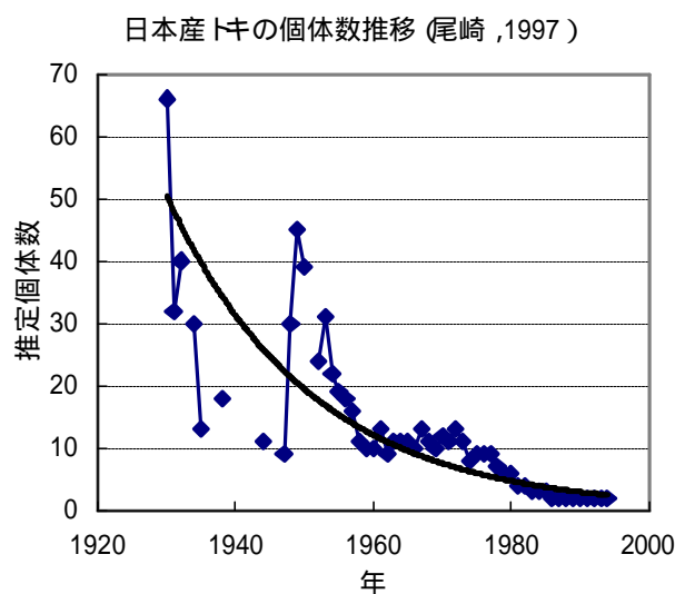
図1. 日本産トキの個体数推移（尾崎，1997）
