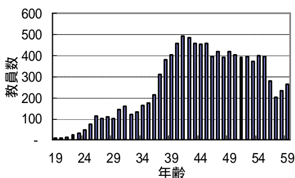
図4. 東京都の高校教員年齢別分布(平成15年度)。40歳以上の中高年教員の割合が高いことが一目でわかる。この年齢別分布を全国のスタンダードと仮定して教員数推移計算を行う。
