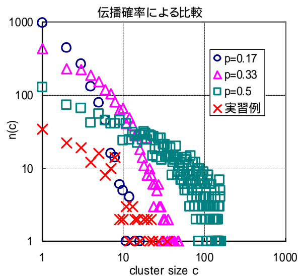
図9. PCによる碁石モデルの仮想地震規模-個数分布(○, △, □)と,プリント実習の仮想地震規模(×). 実習の伝播確率は本文中にもあるように1/3である。PCによる計算では,確率が上がるほど,大規模な地震が増えていることがわかる。またその並び方は大塚(1971)が指摘したように両対数グラフで上に凸となりG-R則とは完全には一致しない(岡本,1997より)。
