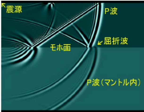
図6．2層構造モデル(モホ面モデル)での地震波伝播のシミュレーション。図で左上隅(地表面)にある爆発震源からのP波とSV波の伝播を地殻とマンテルの弾性定数と密度を境界条件として計算。モホ面から下のマンテル内に地殻内に先駆する波が現れ、それから地表に帰還する屈折波(Head Waveと呼ばれる)が発現するのがわかる。
